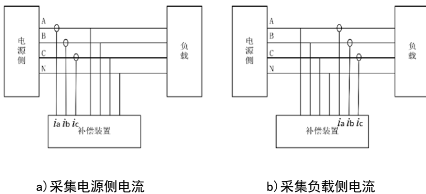
图A.3 装置与三相四线制系统的接线示意图
