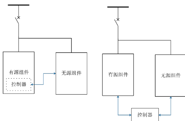
a) 控制器集成于有源组件内
